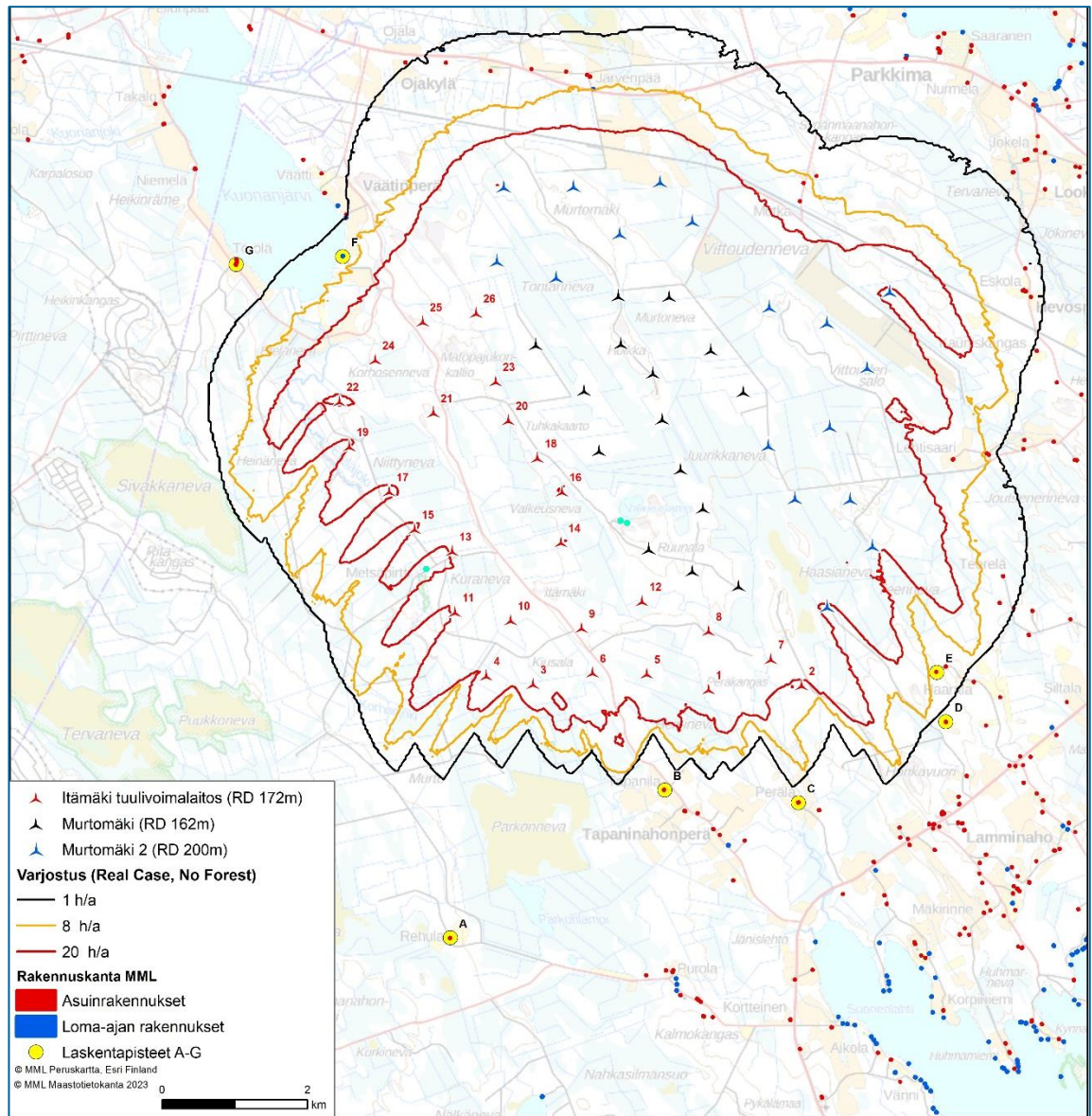
Kuva 6. Varjostuksen yhteismallinnuksen tulos (puuston suojaavaa vaikutusta ei ole huomioitu). Kaava-alueen ne lomarakennukset, jotka kunnan tietojen mukaan ovat todellisuudessa muussa käytössä, on merkitty turkoosilla värillä
