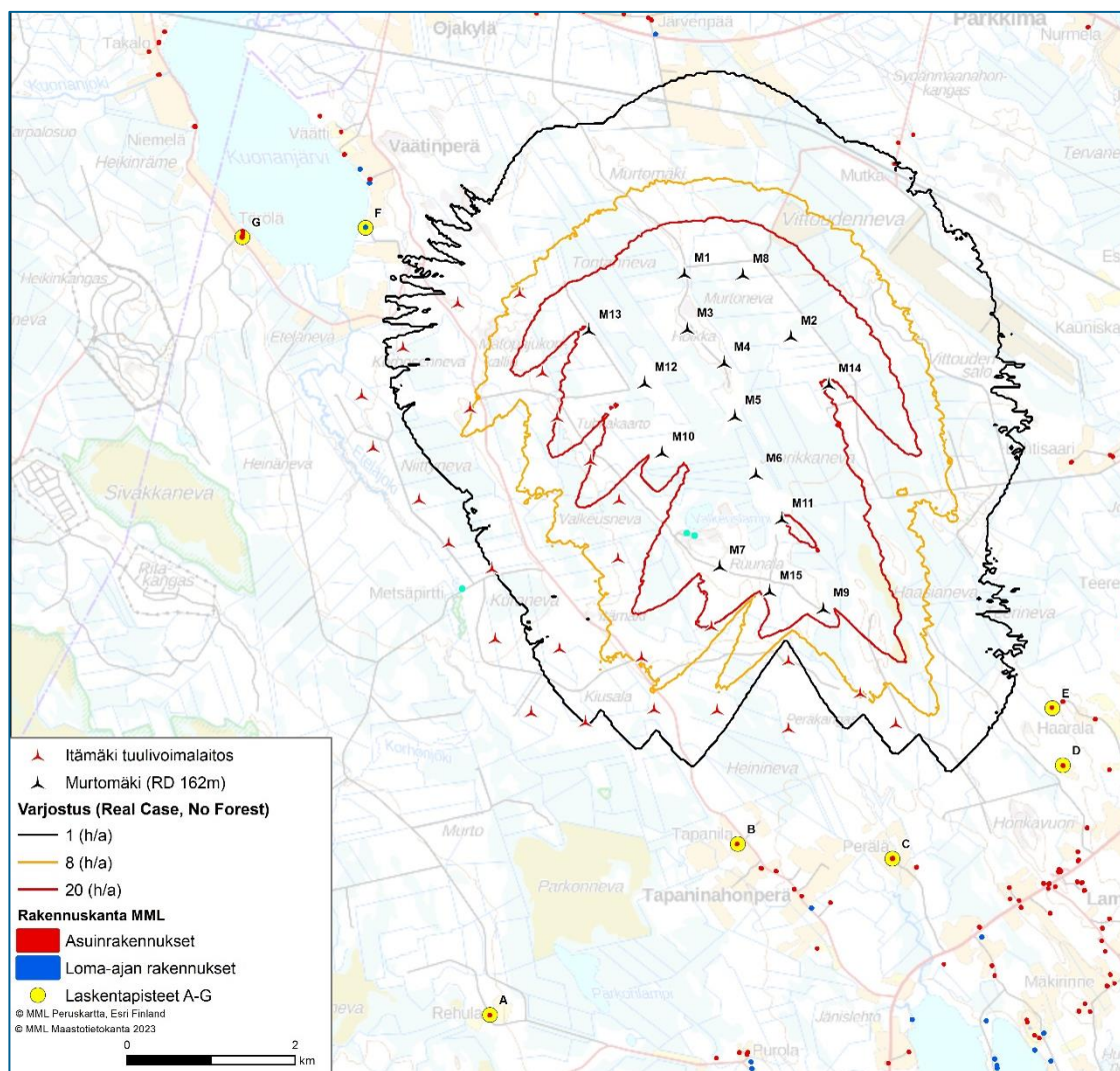
Kuva 3. Laskennalliset varjostusmallinnuksen tulokset nykytilanteessa. Mallinnus on tehty todellisen tilanteen mukaan ilman puuston suojavaikutusta. Kaava-alueen ne lomarakennukset, jotka kunnan tietojen mukaan ovat todellisuudessa muussa käytössä, on merkitty turkoosilla värillä
