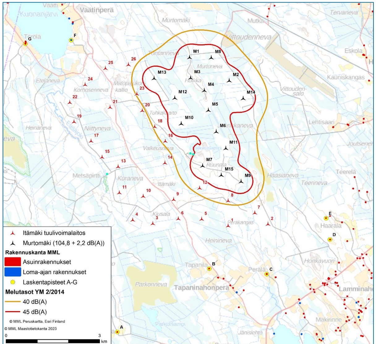
Kuva 1. Laskennalliset Murtomäen tuulivoimatuotannosta aiheutuvat melutasot Itämäen tuulivoimaloiden läheisyydessä nykytilanteessa standardin ISO 9613-2 mukaisesti. Kaava-alueen ne lomarakennukset, jotka kunnan tietojen mukaan ovat todellisuudessa muussa käytössä, on merkitty turkoosilla värillä
