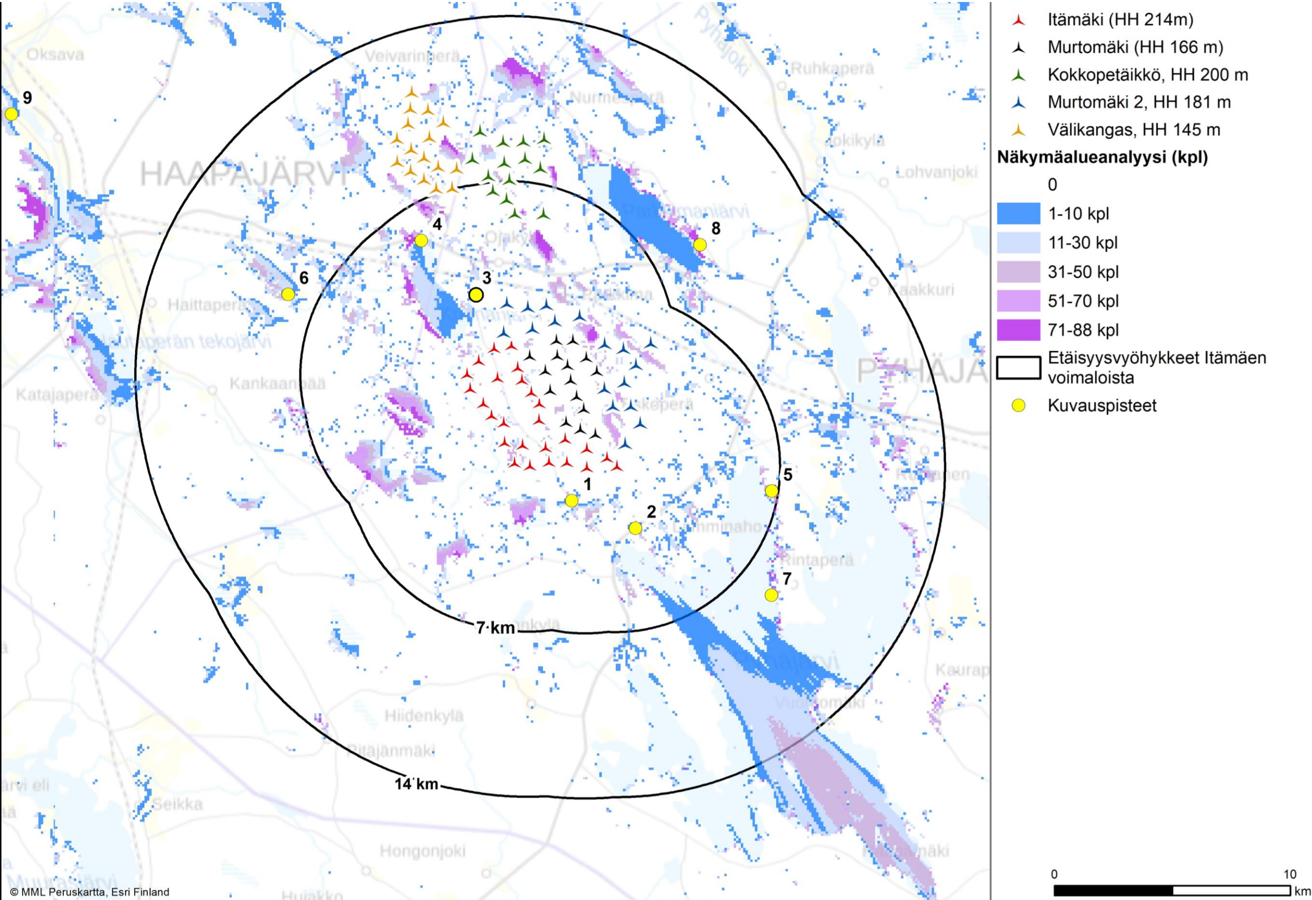
Kuva 1b. Itämaen, Murtomäki 2:n, Kokkopetäikön ja Välikankaan tuulivoimahankkeiden sekä Murtomäen tuulivoimapuiston näkymäalueanalyysin laskentatulokset voimaloiden napakorkeudella mallinnettuna.
