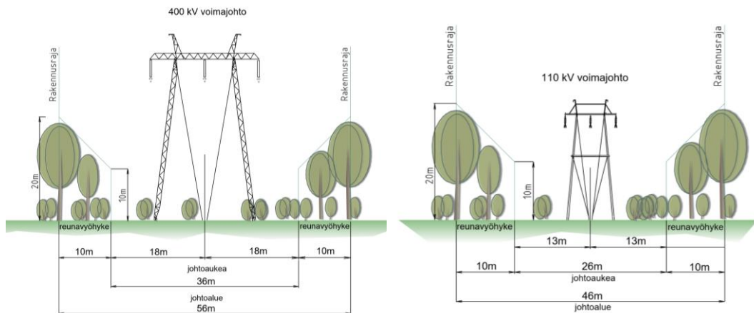
Kuva 2-17. Voimajohtoalueen poikkileikkaus ja voimajohdon vaatima maa-ala. Vasemmalla on 110 kV voimajohto ja oikealla 400 kV voimajohto.
