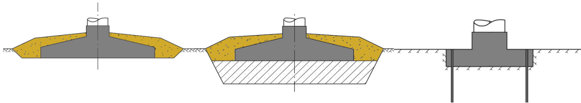
Kuva 2-15. Tuulivoimalat voidaan perustaa useilla eri tavoilla. Periaatekuvat maavaraisesta teräs- betoniperustuksesta, teräsbetoniperustuksesta massanvaihdon sekä kallioankku- roidusta teräsbetoniperustuksesta.
